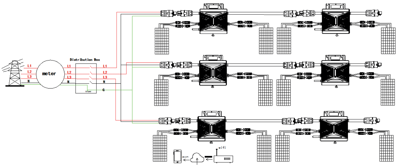
Schéma d'une connexion parallèle triphasée
