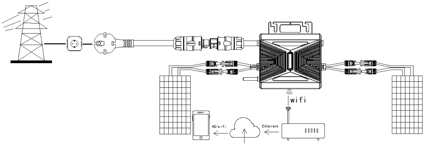
Schéma de câblage de la version autonome
