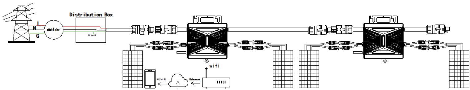
Schéma de connexion parallèle monophasée
